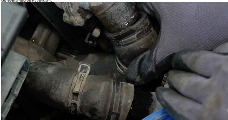
Vahetamine: termostaat - VAUXHALL Astra Mk1 Kombi. AUTODOC soovitab: • Tähelepanu! Jahutusvedelik võib lekkida jahutustorust ja termostaadi korpusest.
